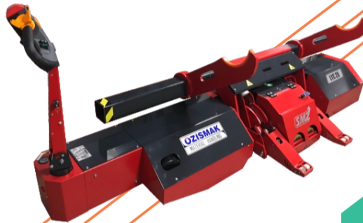
SMZ 4 YÖN HAREKETLİ LEVENT TAŞIYICI
